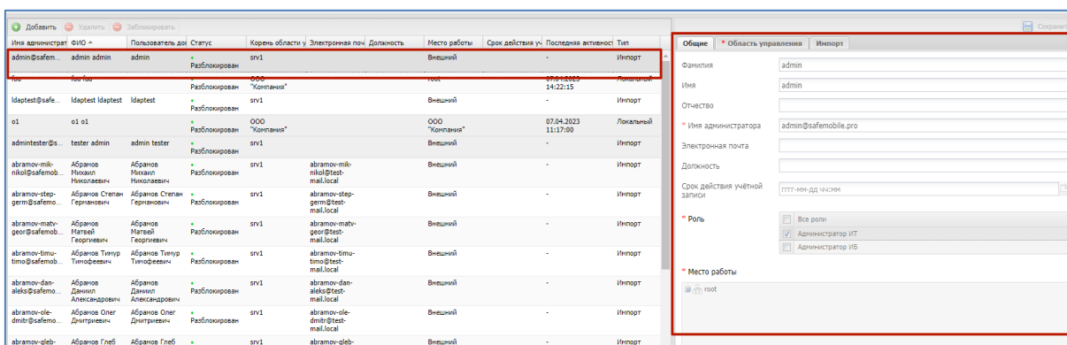
Рисунок 2.107 - Окно «Администратор»
