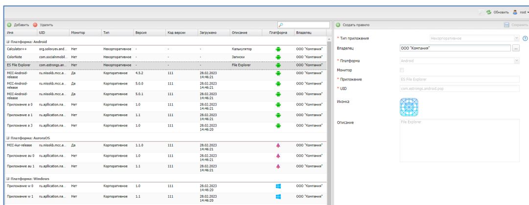
Рисунок 2.114 - Окно «Приложения»
