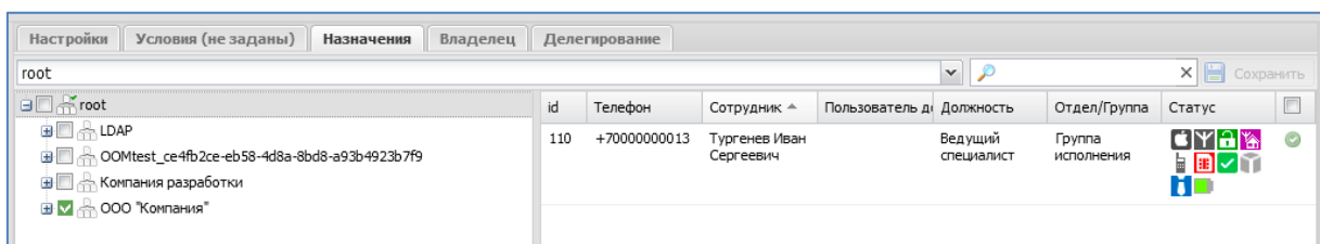
Рисунок 2.64 - Назначение ПУП
