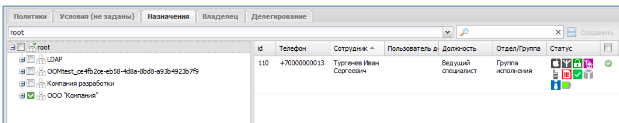
Рисунок 2.51 - Назначение профиля
