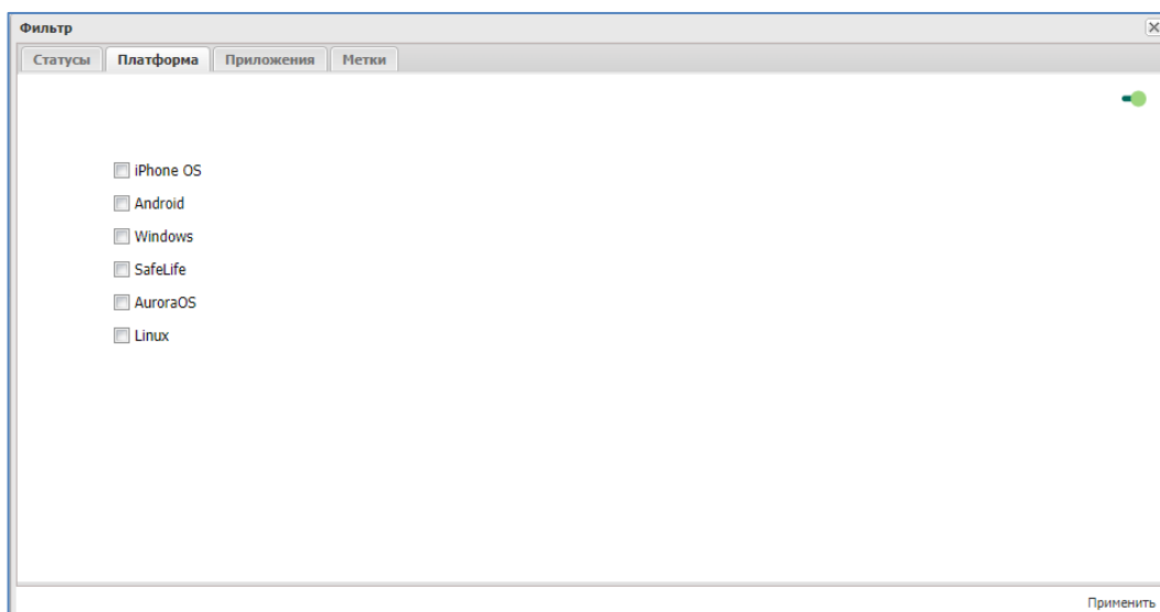
Рисунок 2.13 - Вкладка «Платформа»
