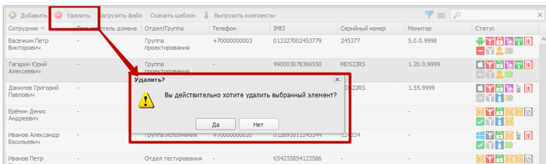
Рисунок 2.130 - Удаление комплекта
