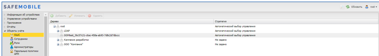
Рисунок 2.95 - Окно «ОШС»
