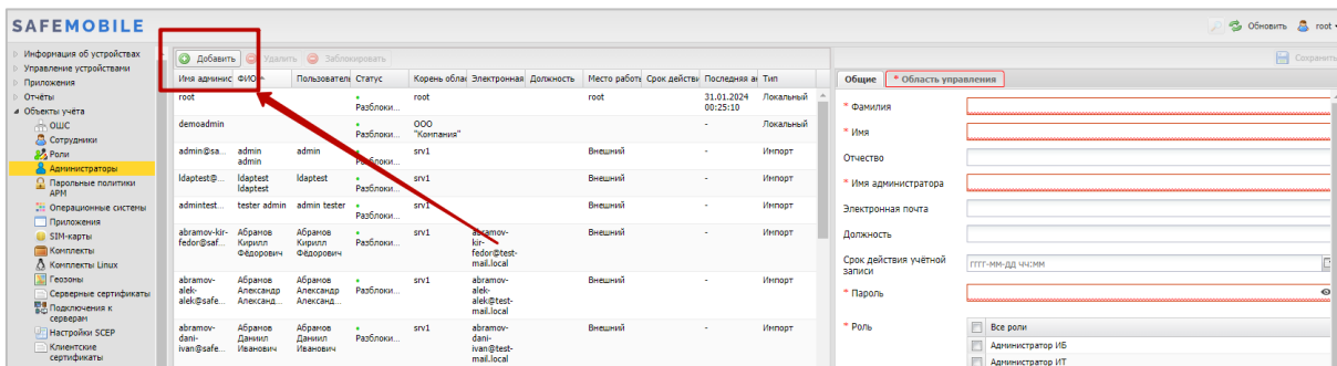
Рисунок 2.108 - Создание Администратора
