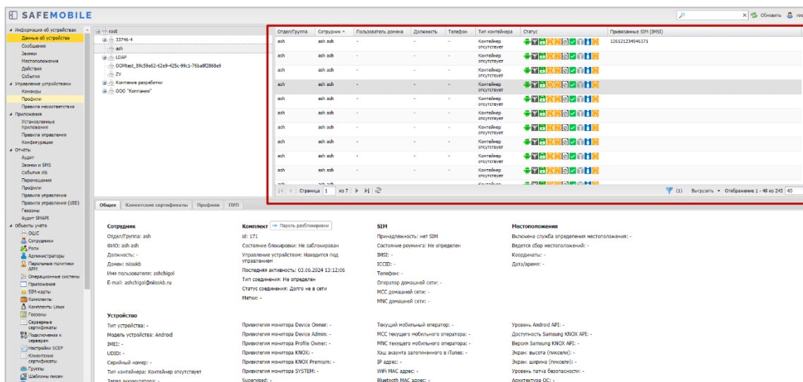
Рисунок 2.18 - Главная таблица
