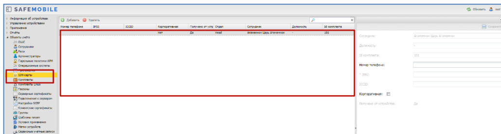
Рисунок 2.121 - Окно SIM-карты
