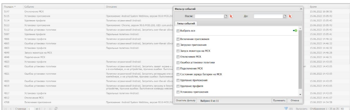
Рисунок 2.42 - Фильтрация событий
