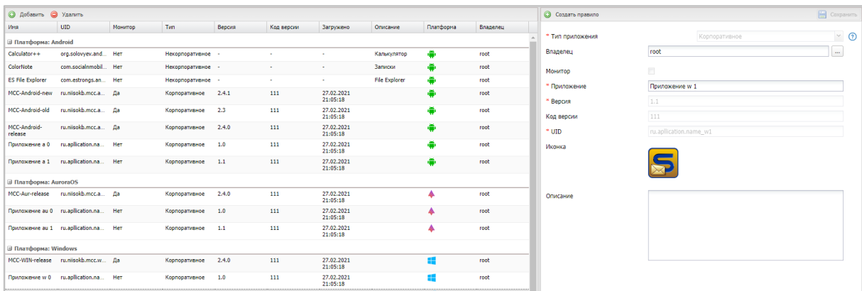
Рисунок 2.119 - Редактирование приложения
