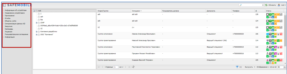
Рисунок 2.20 - Главное меню
