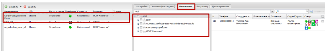
Рисунок 2.73 - Назначение конфигурации
