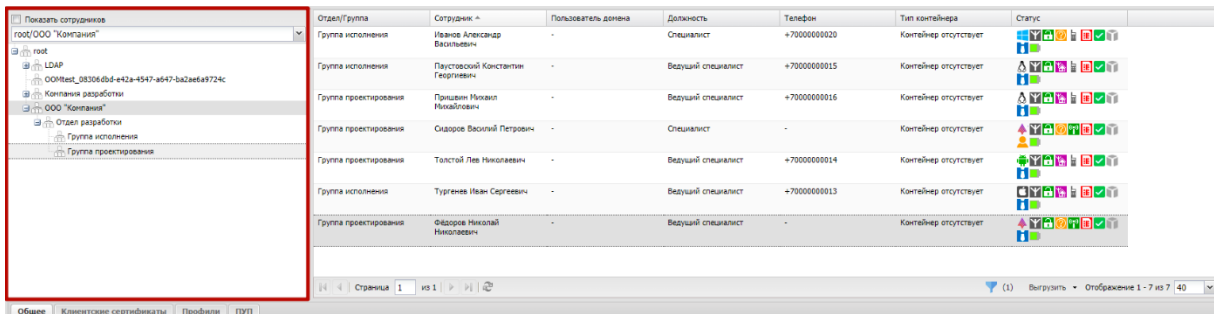
Рисунок 2.15 - Панель ОШС
