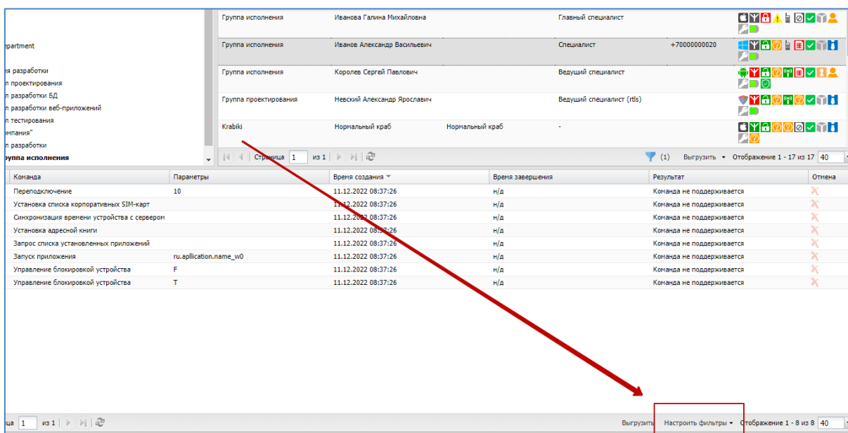
Рисунок 2.40 - Фильтрация действий
