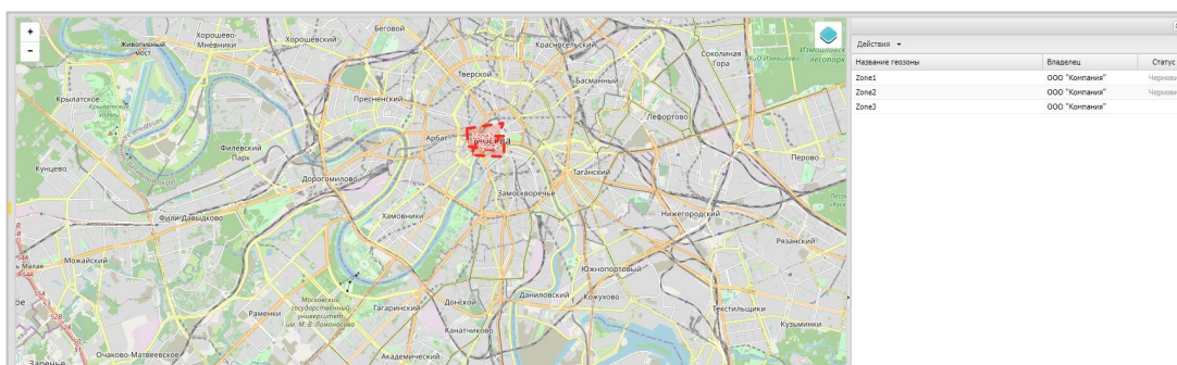
Рисунок 2.135 - Окно «Геозоны»
