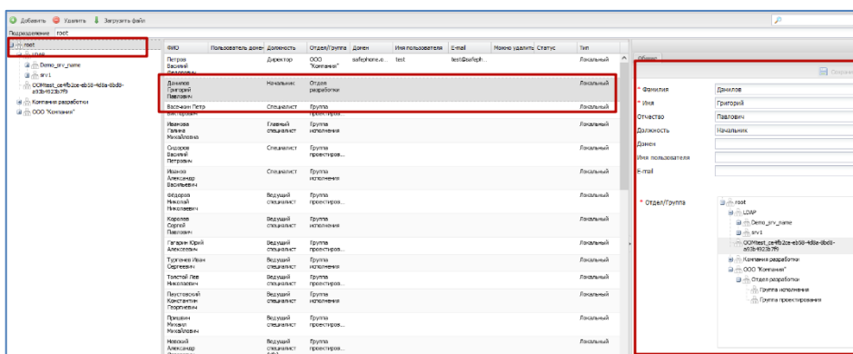
Рисунок 2.99 - Окно «Сотрудник»
