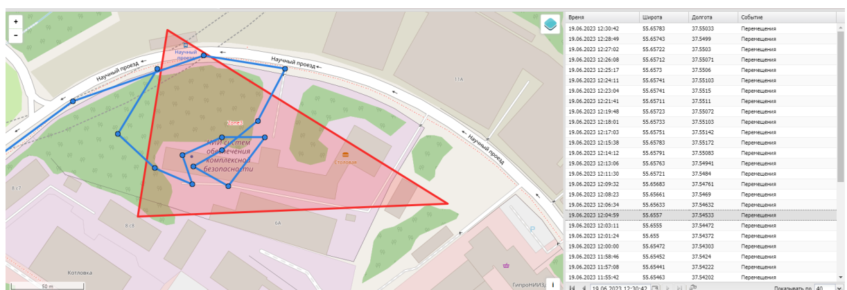
Рисунок 2.35 - Раздел «Местоположения»
