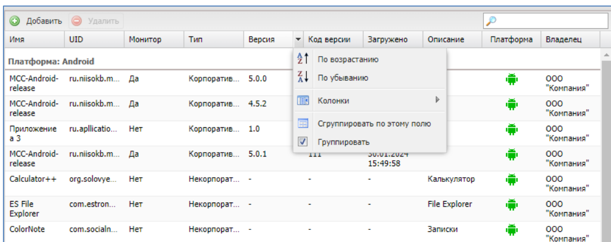
Рисунок 2.115 - Группировка приложений
