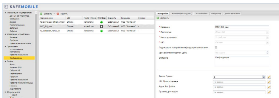
Рисунок 2.68 - Окно «Конфигурации»
