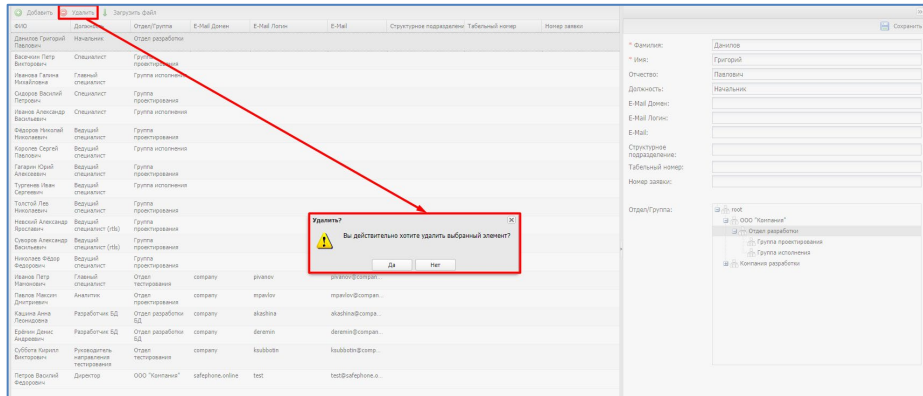
Рисунок 2.101 - Удаление сотрудника
