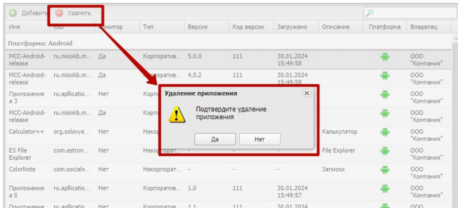
Рисунок 2.120 - Удаление приложения
