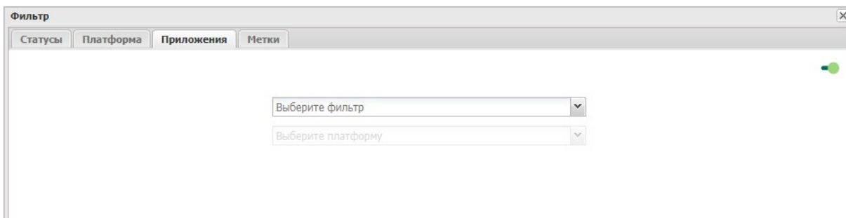
Рисунок 2.14 - Вкладка «Приложения»
