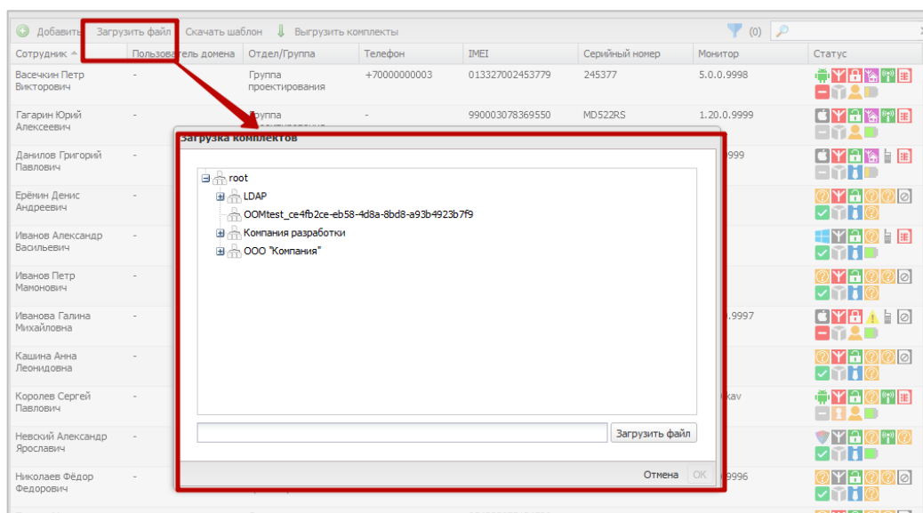
Рисунок 2.127 - Загрузка комплектов
