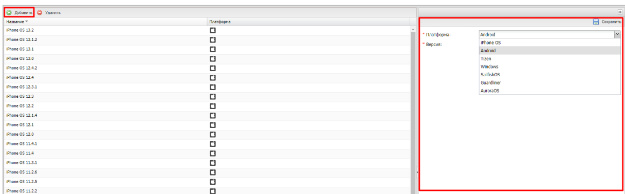
Рисунок 2.112 - Добавление ОС
