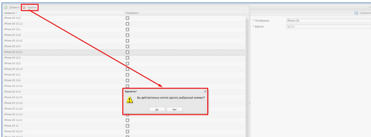
Рисунок 2.113 - Удаление ОС
