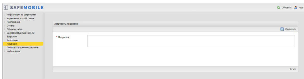
Рисунок 2.196 - Окно «Лицензия»
