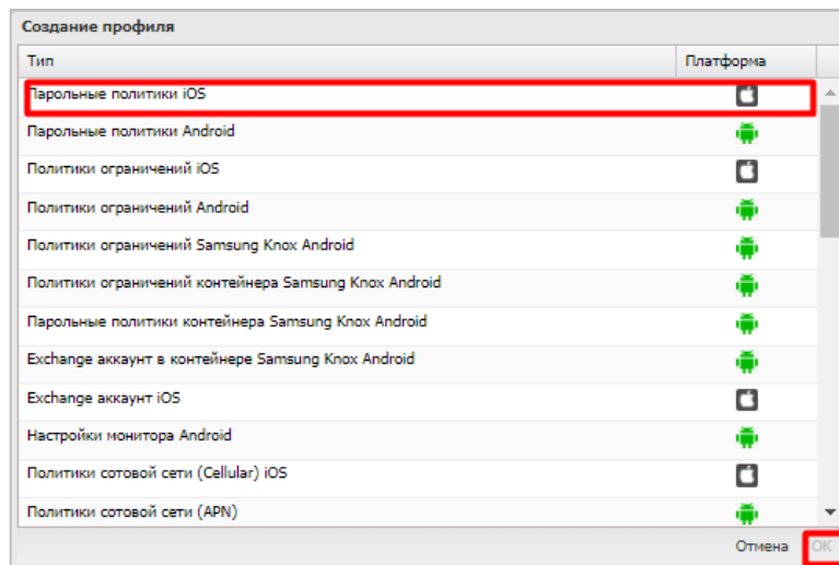
Рисунок 2.48 - Создание профиля
