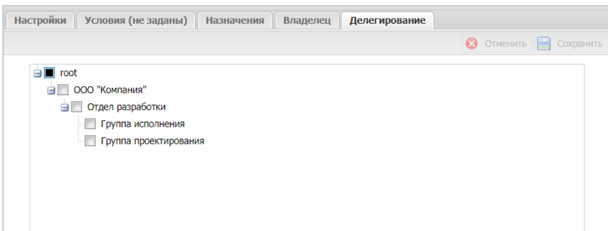
Рисунок 2.66 - Делегирование сущности
