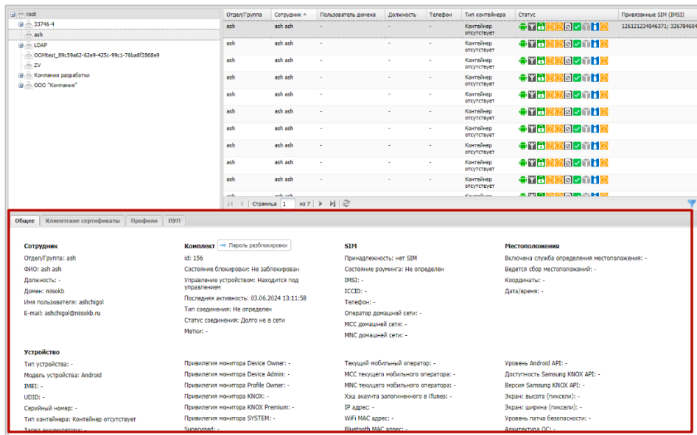
Рисунок 2.19 - Информационная таблица
