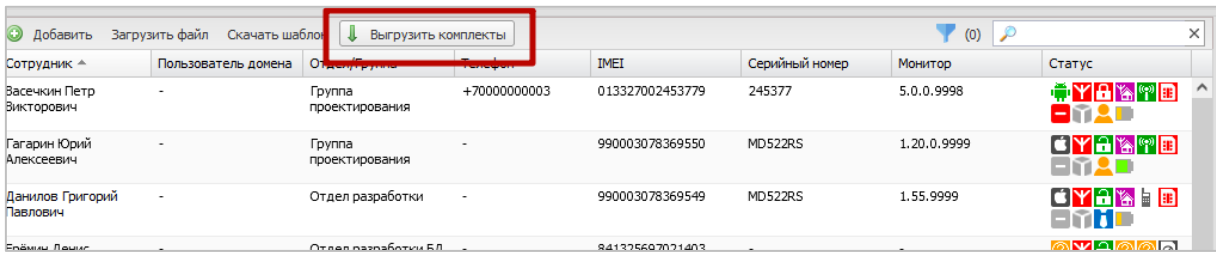
Рисунок 2.128 - Выгрузка комплектов
