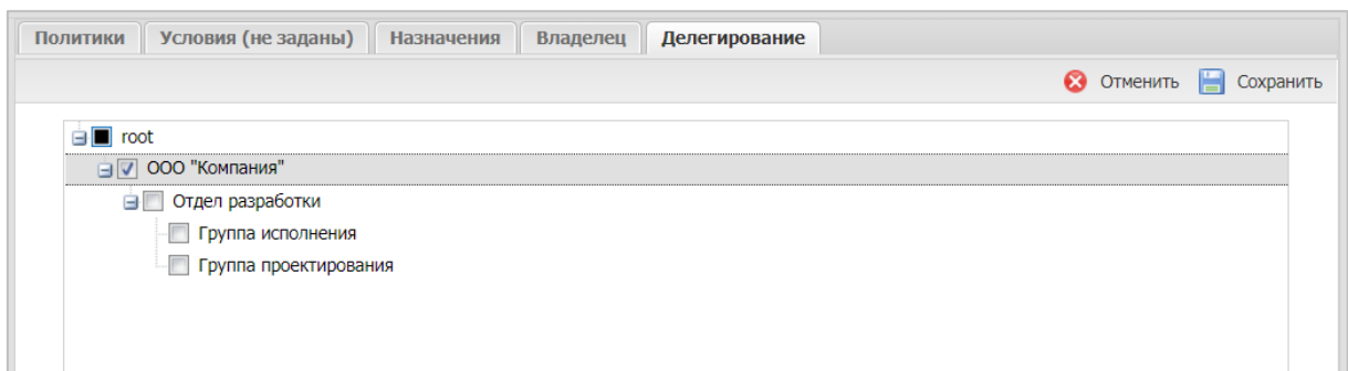
Рисунок 2.54 - Делегирование сущности
