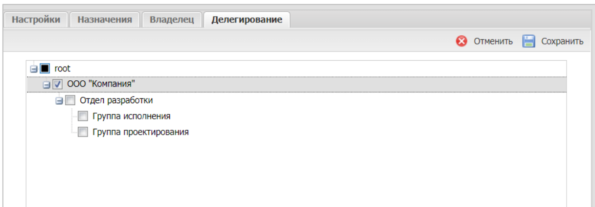
Рисунок 2.75 - Делегирование сущности
