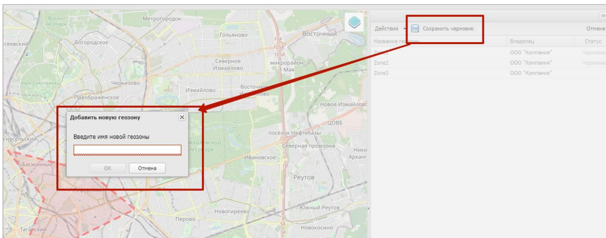
Рисунок 2.137 - Добавление геозоны
