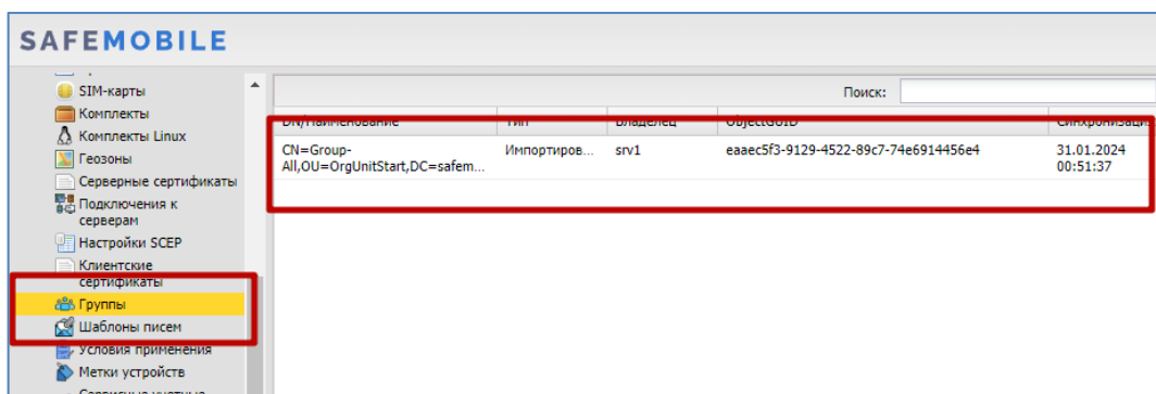
Рисунок 2.150 - Список групп
