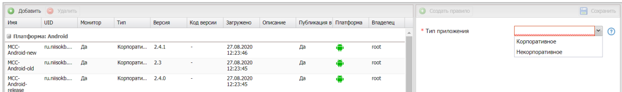
Рисунок 2.116 - Добавление приложения
