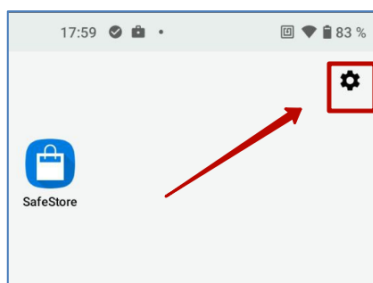
Рисунок 44 – Кнопка «Настройки»
