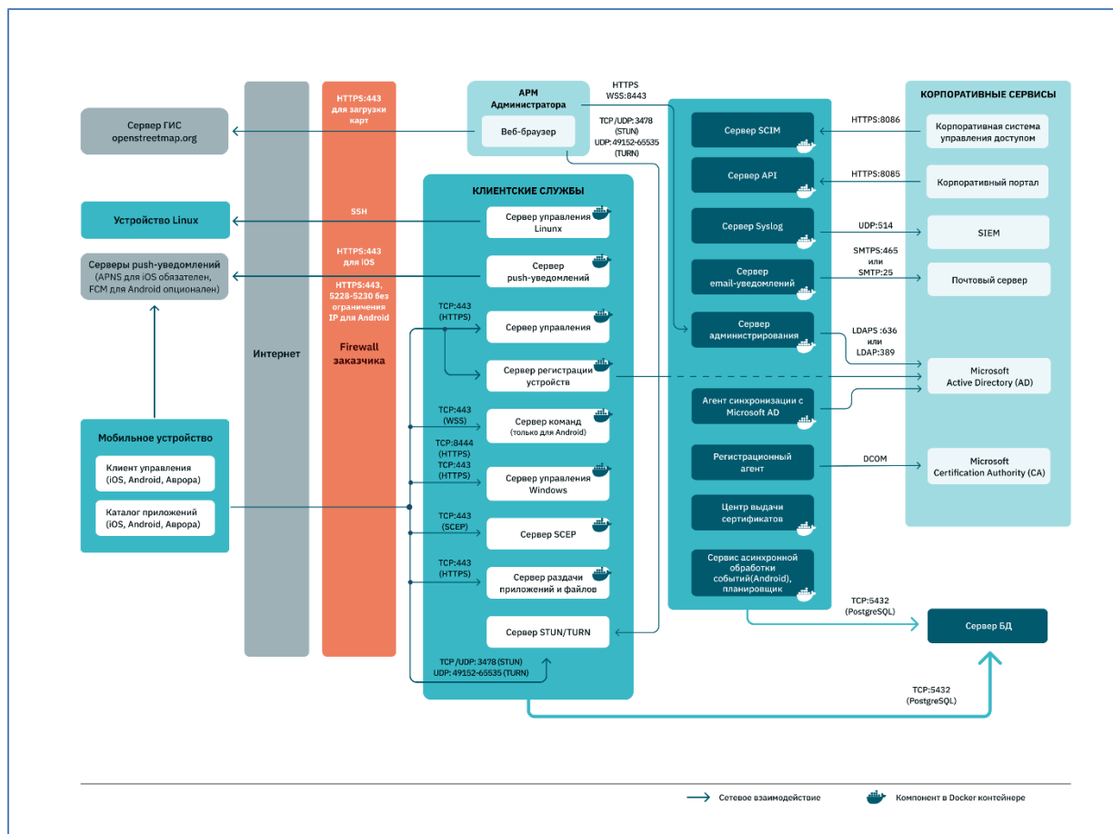
Рисунок 1.1 — Архитектурная схема
