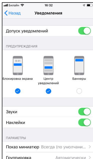
Рисунок 30 – Настройка уведомлений
