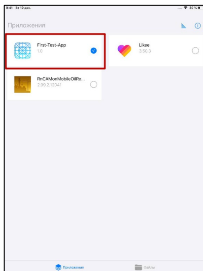
Рисунок 40 – Установленное приложение
