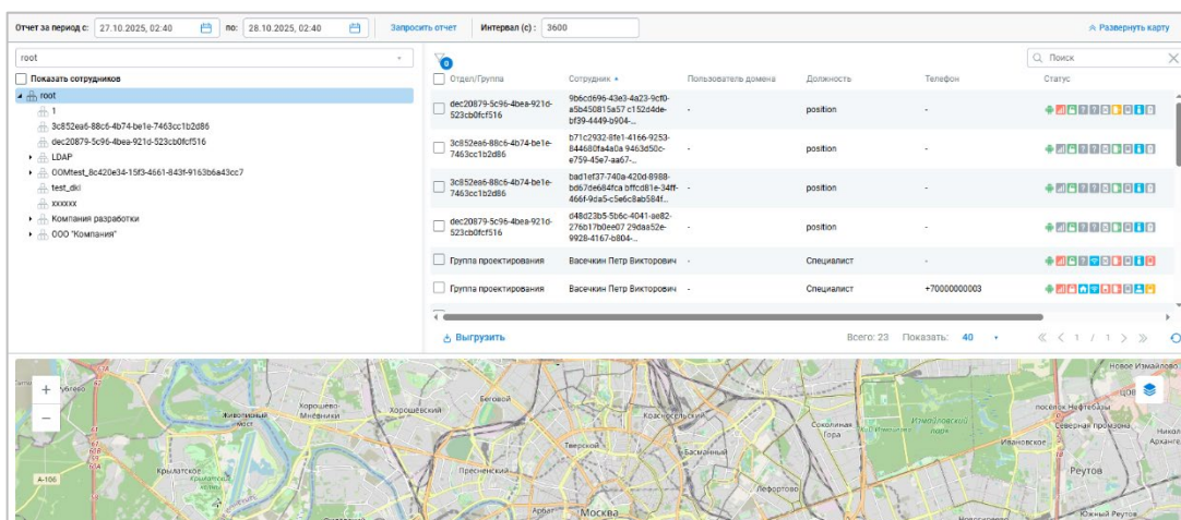
Рисунок 2.101 — Окно «Перемещения»
