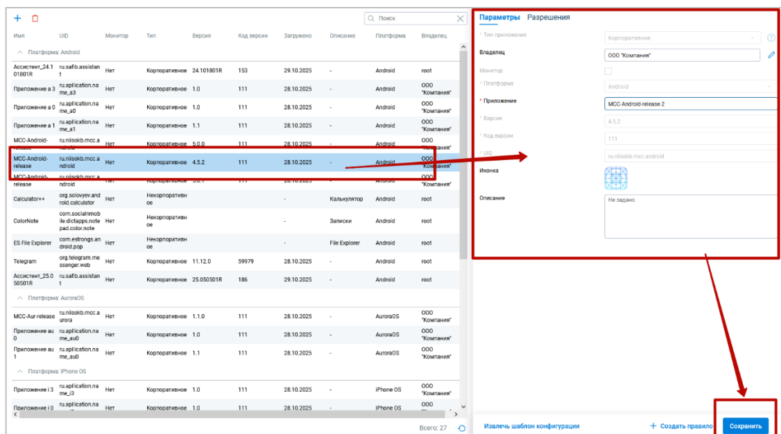
Рисунок 2.135 — Редактирование приложения
