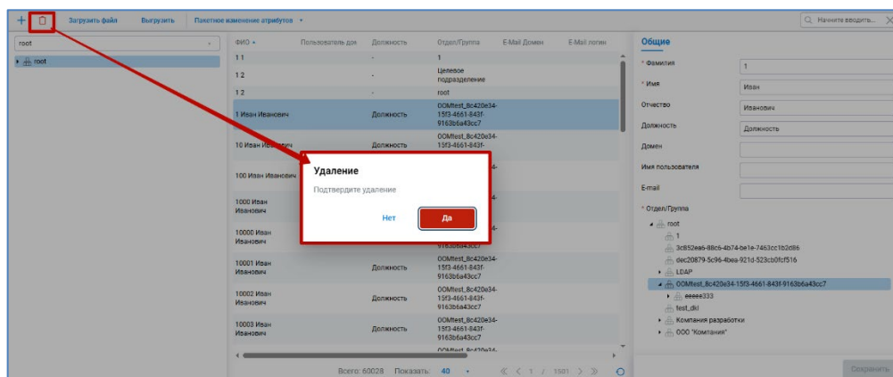
Рисунок 2.115 — Удаление сотрудника
