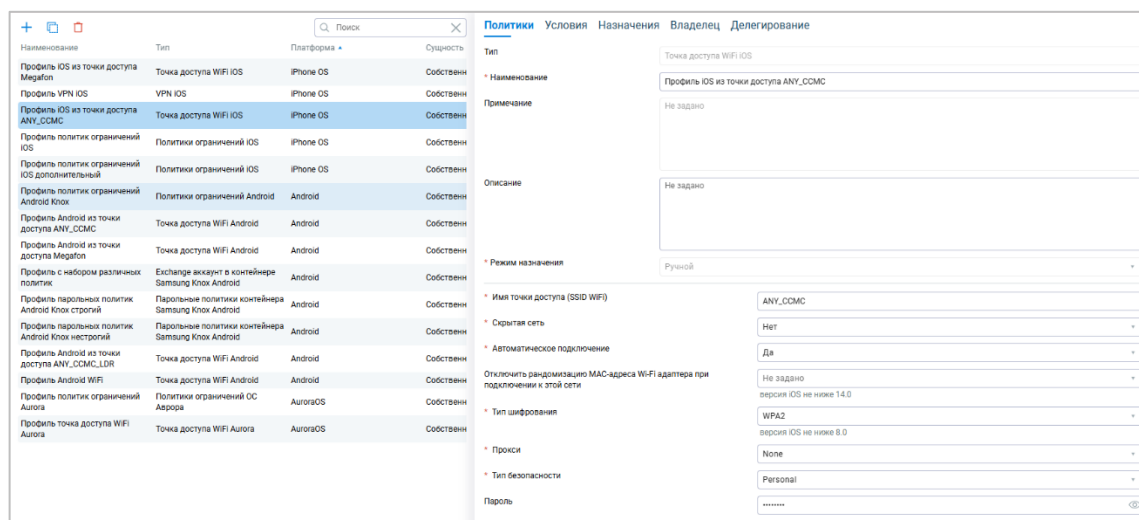
Рисунок 2.54 — Окно «Профили»
