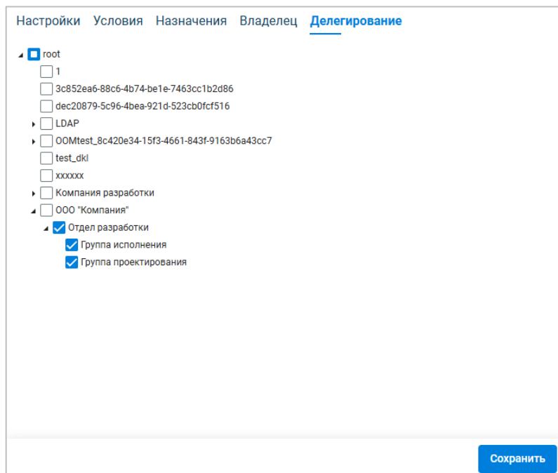
Рисунок 2.94 — Делегирование сущности
