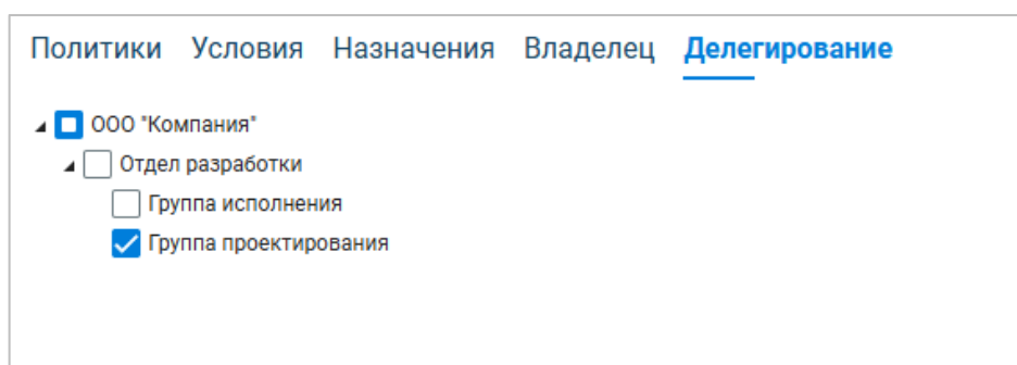
Рисунок 2.62 — Делегирование сущности
