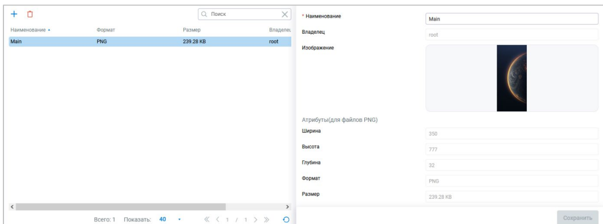
Рисунок 2.179 — Раздел «Файлы»
