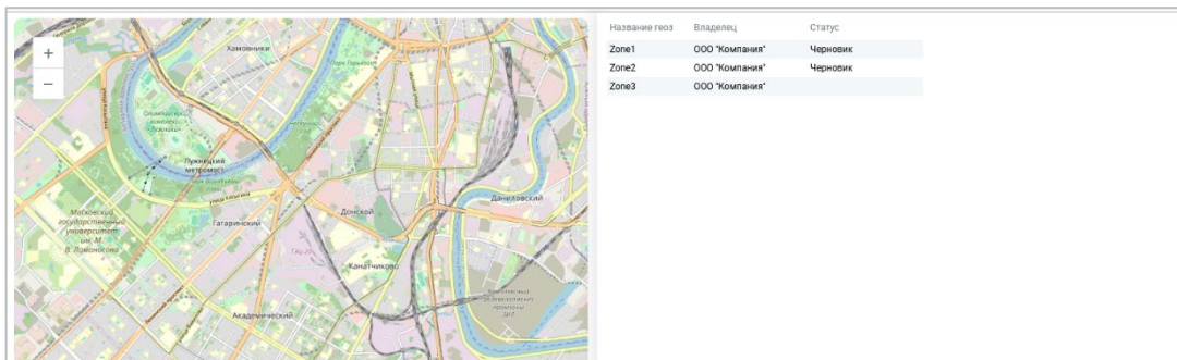
Рисунок 2.154 — Окно «Геозоны»
