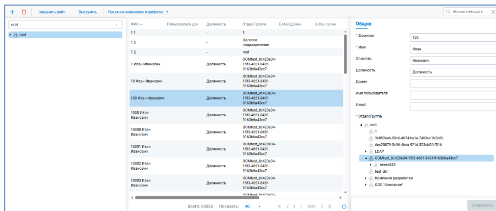
Рисунок 2.113 — Окно «Сотрудник»
