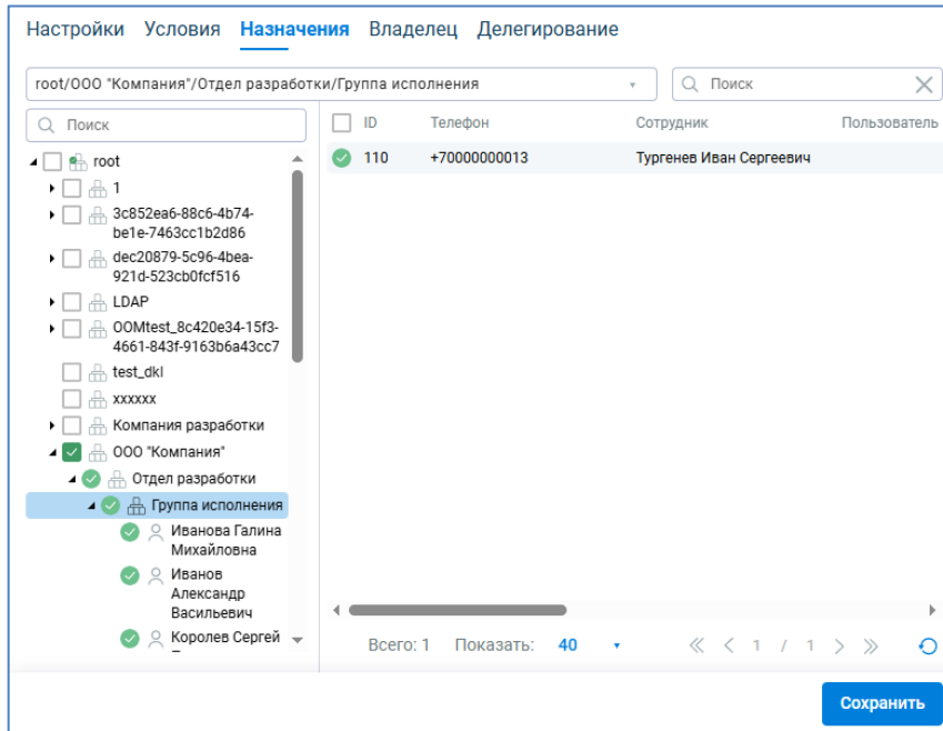
Рисунок 2.82 — Назначение ПУП
