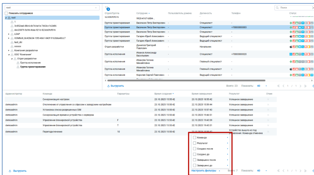
Рисунок 2.46 — Фильтрация действий
