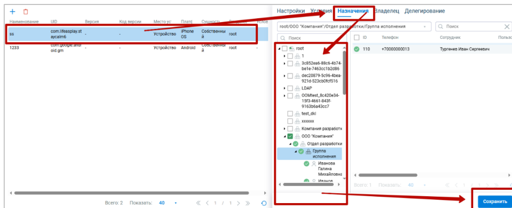
Рисунок 2.92 — Назначение конфигурации
