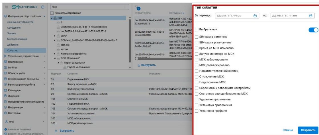
Рисунок 2.48 — Фильтрация событий
