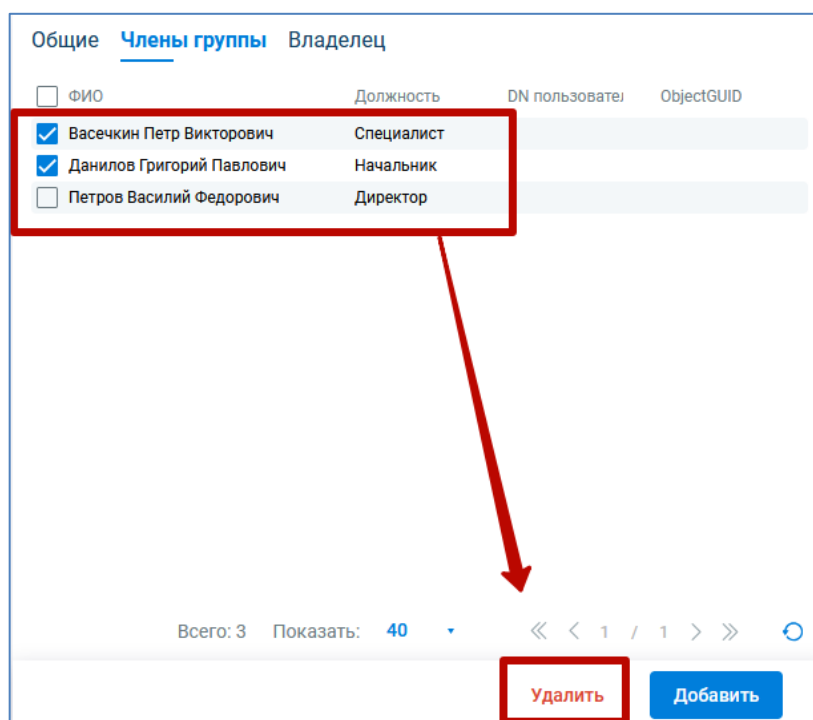
Рисунок 2.171 — Удаление сотрудника
