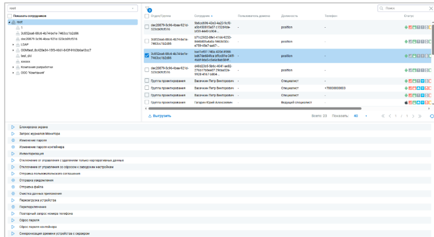
Рисунок 2.50 — Раздел «Команды»
