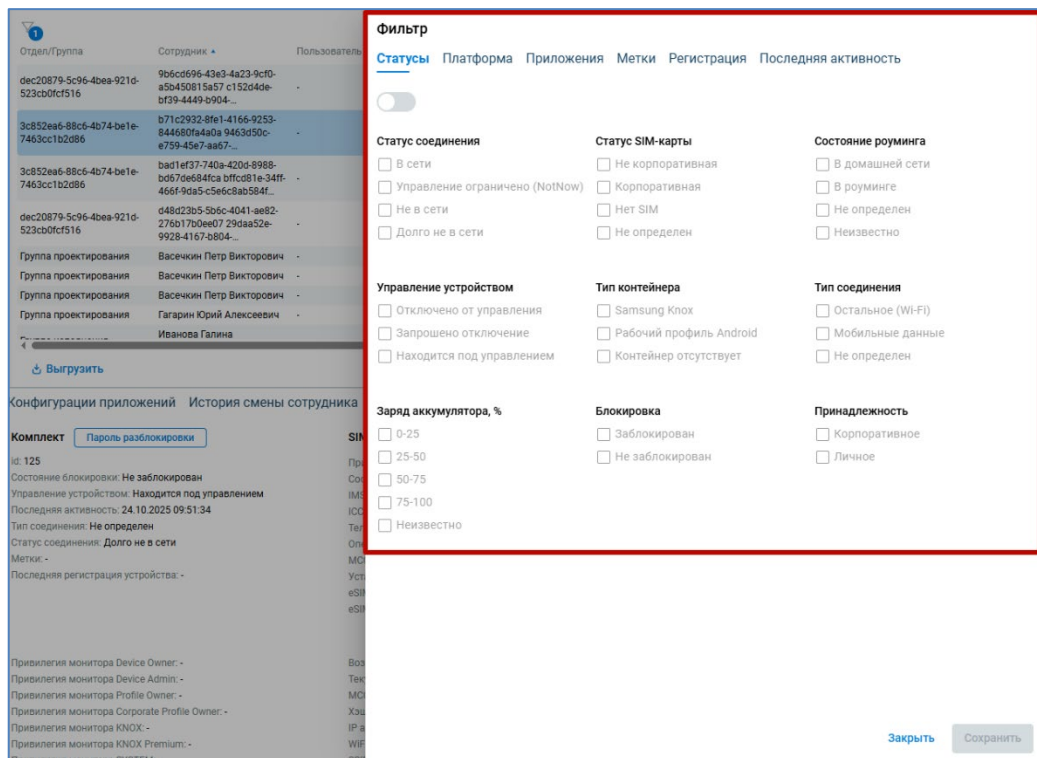
Рисунок 2.13 — Вкладка «Статусы»
