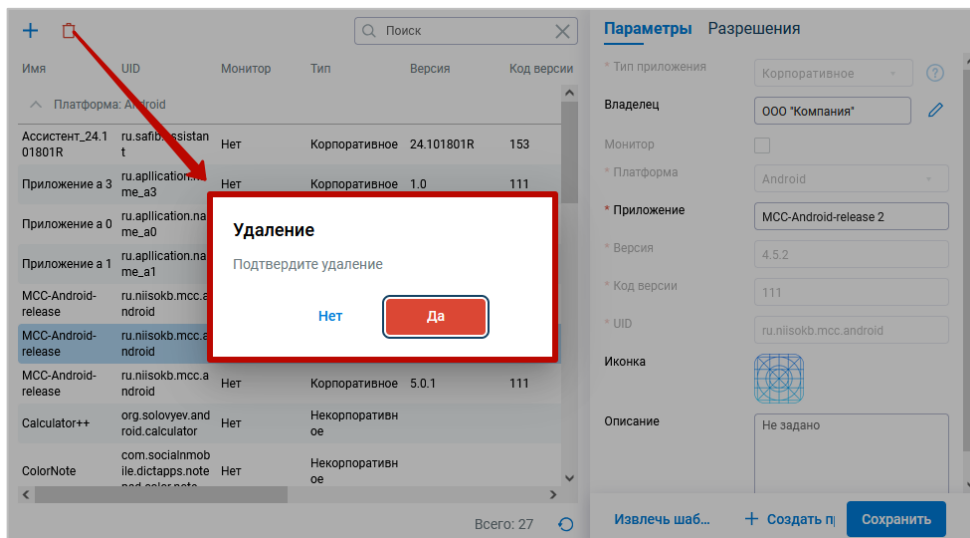
Рисунок 2.136 — Удаление приложения
