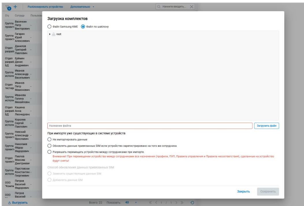
Рисунок 2.144 — Загрузка комплектов
