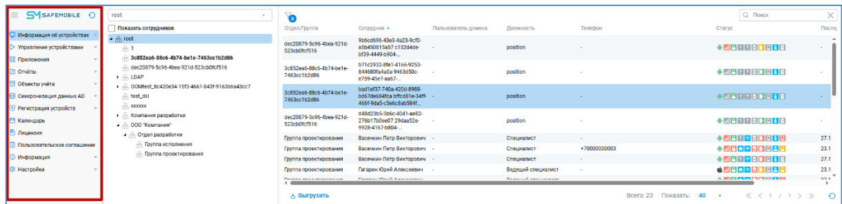
Рисунок 2.26 — Главное меню
