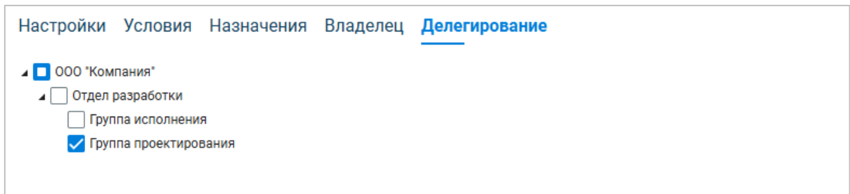
Рисунок 2.84 — Делегирование сущности
