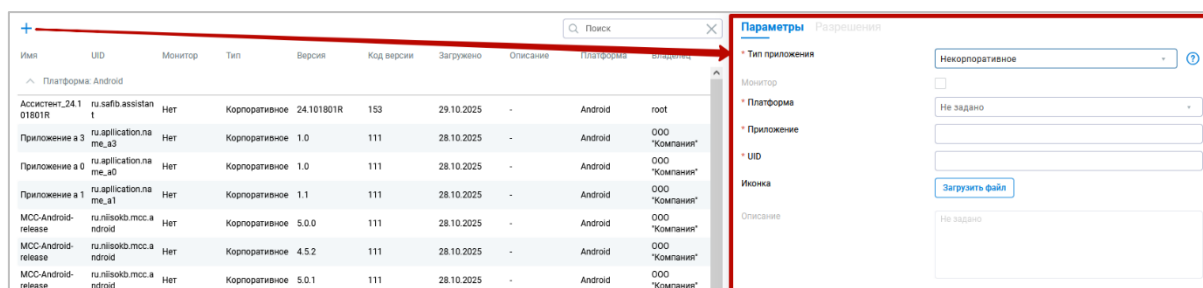
Рисунок 2.132 — Добавление приложения
