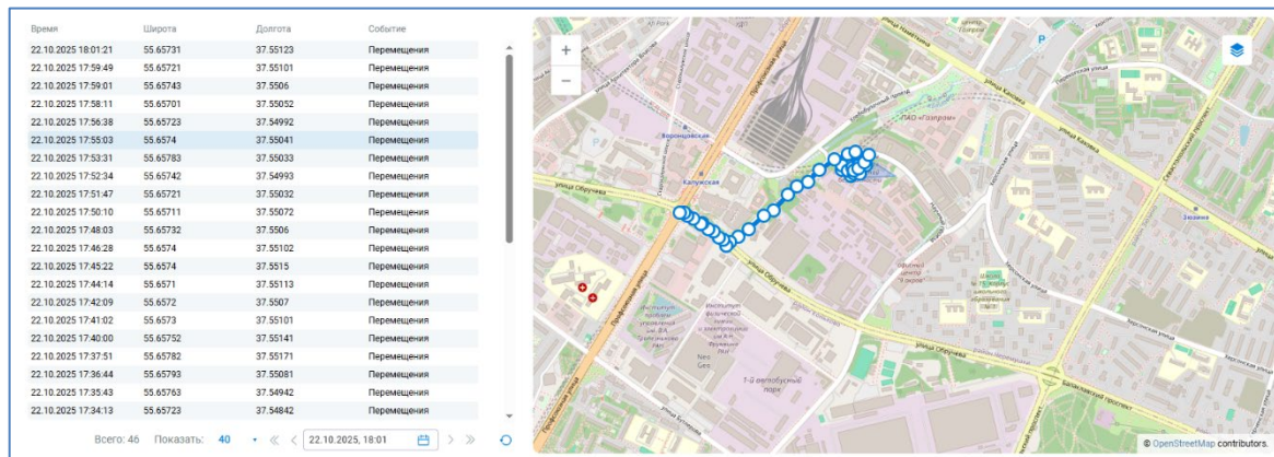
Рисунок 2.41 — Раздел «Местоположения»
