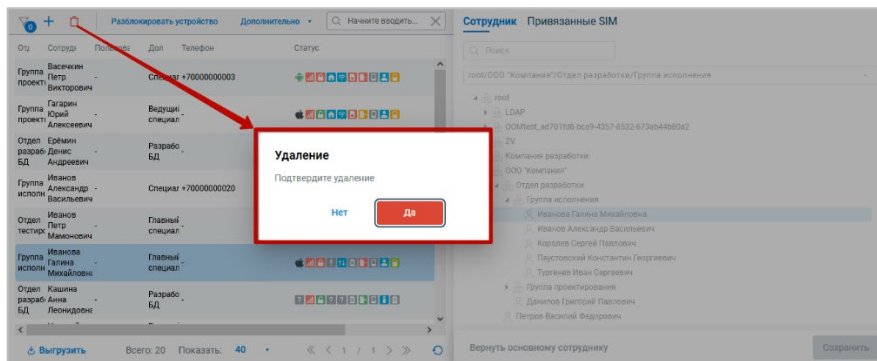
Рисунок 2.147 — Удаление комплекта
