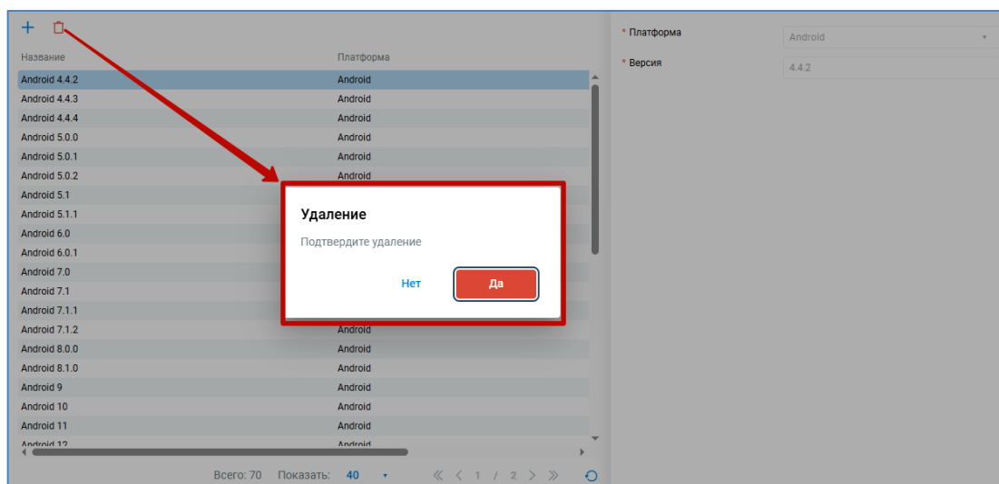
Рисунок 2.130 — Удаление ОС
