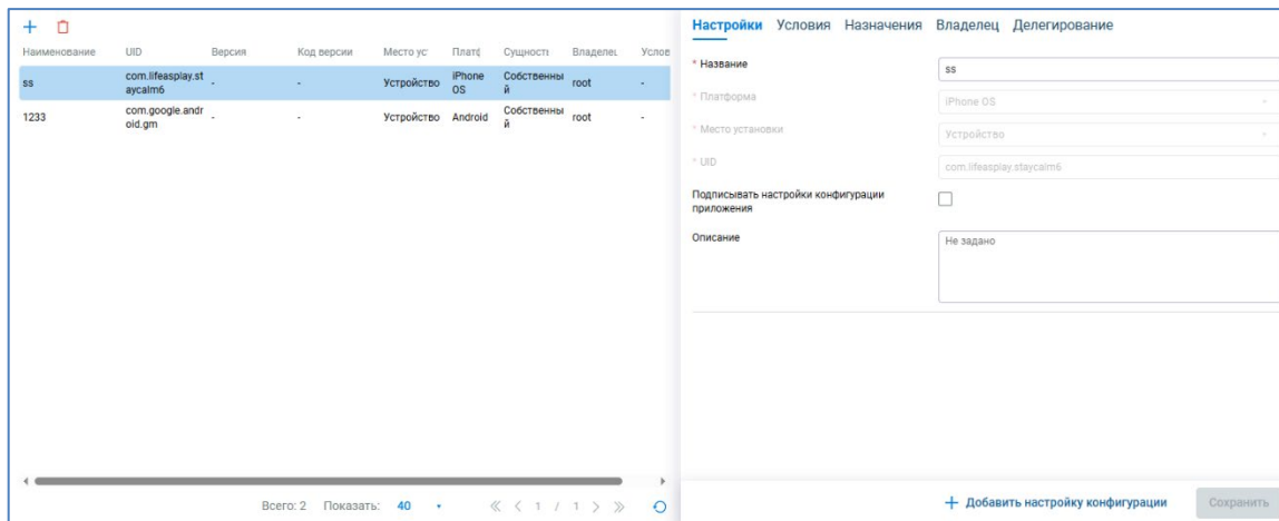
Рисунок 2.87 — Окно «Конфигурации»
