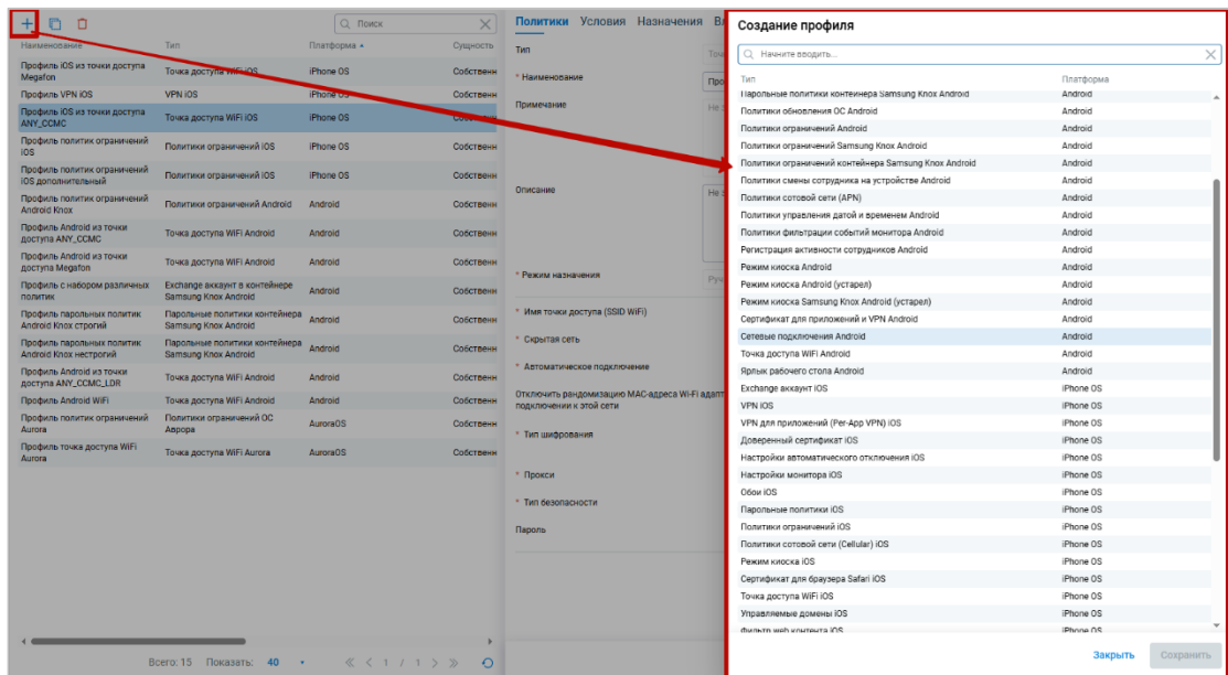
Рисунок 2.55 — Создание профиля
