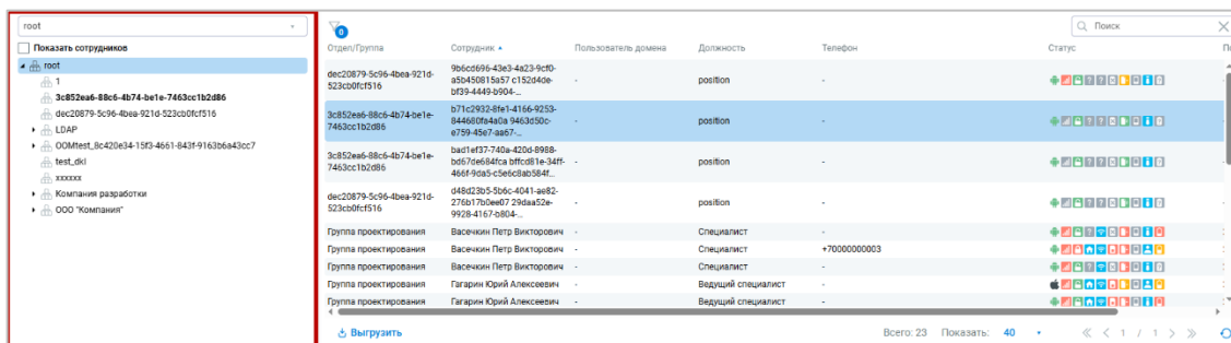
Рисунок 2.19 — Панель ОШС
