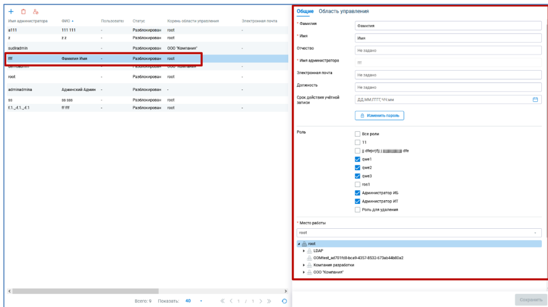
Рисунок 2.123 — Окно «Администратор»
