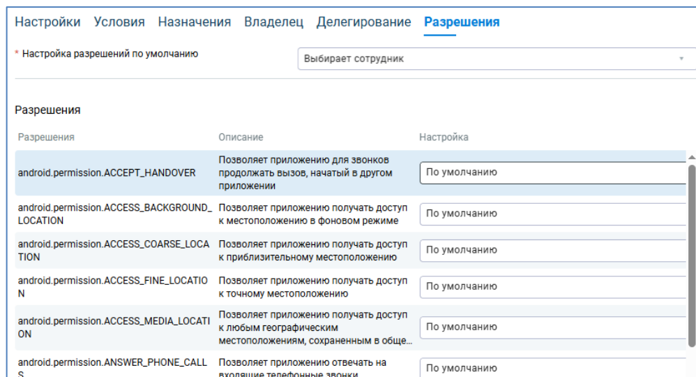
Рисунок 2.85 — Вкладка «Разрешения»
