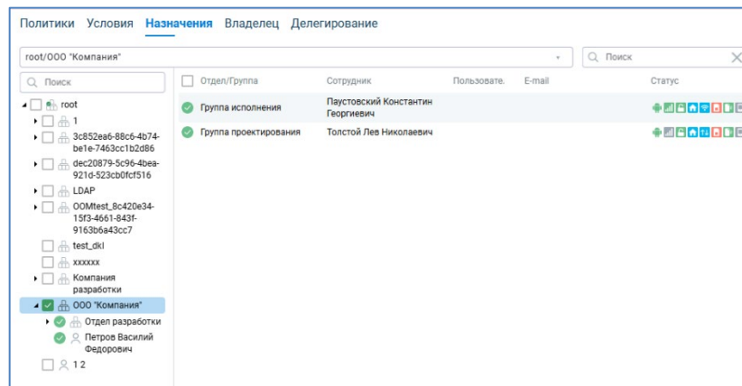
Рисунок 2.59 — Назначение профиля
