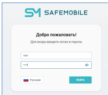
Рисунок 2.1 — Окно аутентификации
