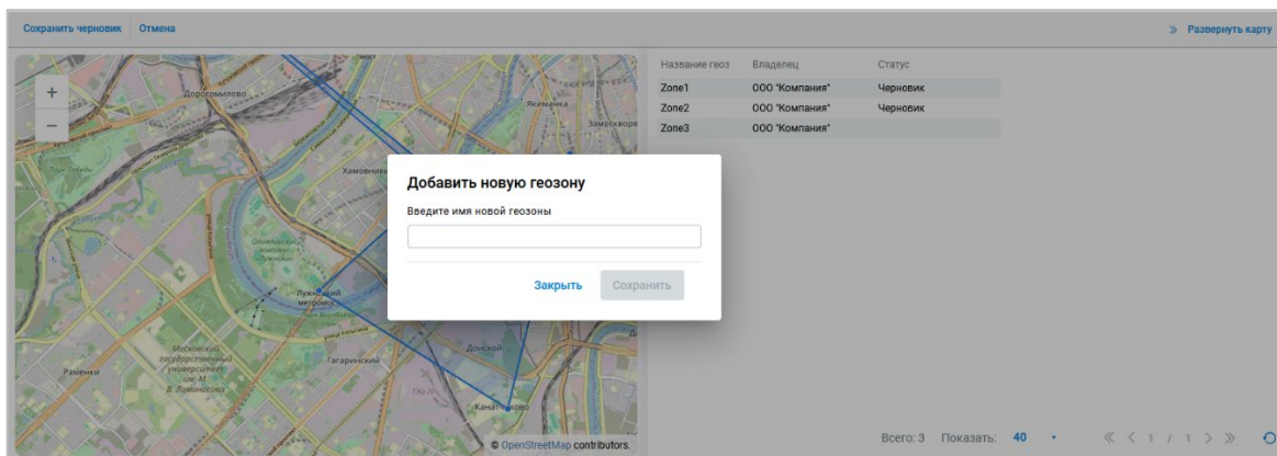
Рисунок 2.155 — Добавление геозоны
