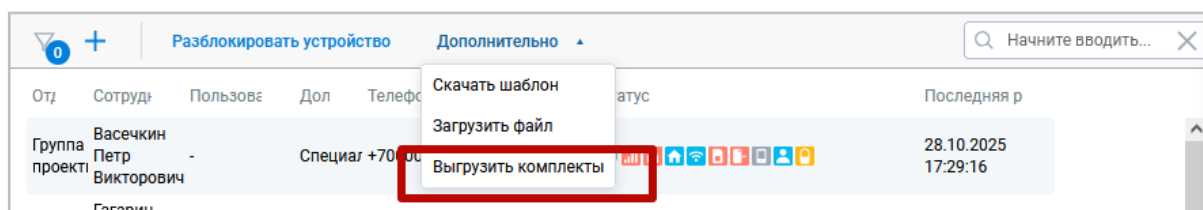
Рисунок 2.145 — Выгрузка комплектов
